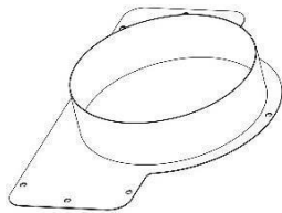
Adaptateur/clapet 6" X 3.25" (Pour évacuation verticale) horizontale)
